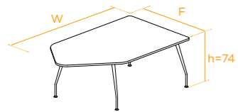
MESA TRAPEZOIDAL T2 DOBLE T2 DOUBLE TRAPEZOIDAL TABLE TABLE TRAPÉZOÏDALE DOBLE T2
